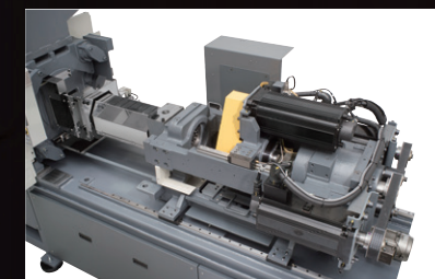
リニアガイド摺動 フリクションフリードライブ Linear guide sliding friction free drive
